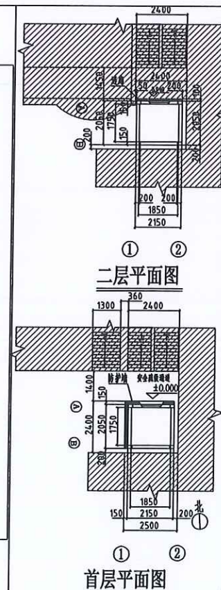
平面图一
