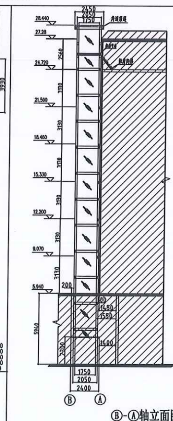
B-A轴立面图
