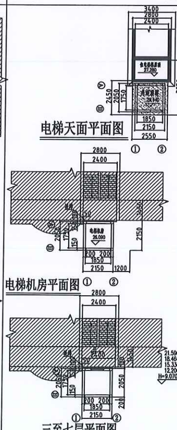
平面图二
